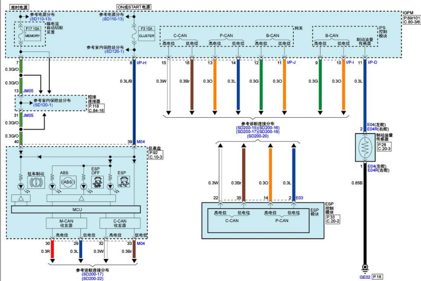
电控稳定程序(ESP)系统(1)
